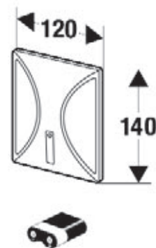
Infrarot-Urinal Elektronik für Batteriebetrieb
